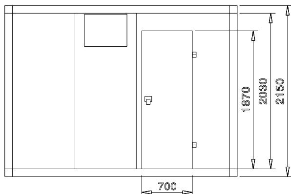
Zepředu
