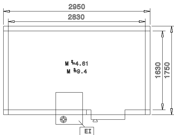
Boční
